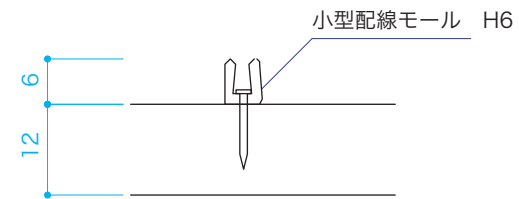
レール部分 S=1/1
