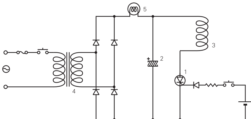
図4-1 マグネカタパルト 回路図
